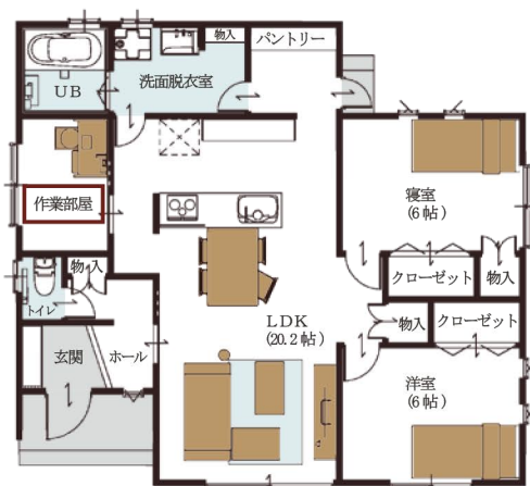
延床面積…79.49㎡ (24.04坪)
