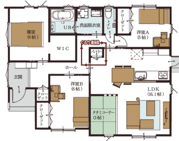
延床面積…86.95㎡ (26.30坪)
